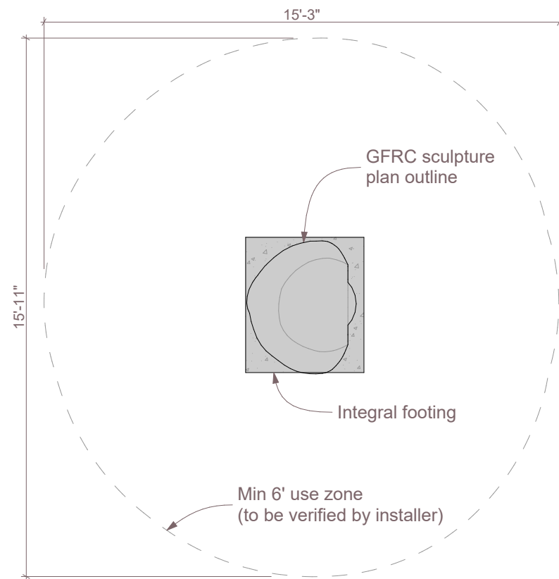
2 Plan SCALE: 1/4" = 1'-0"
