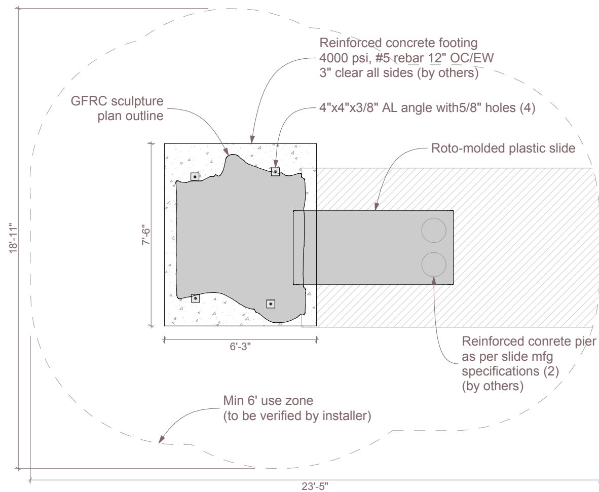
Plan SCALE: 1/4" = 1'-0"
