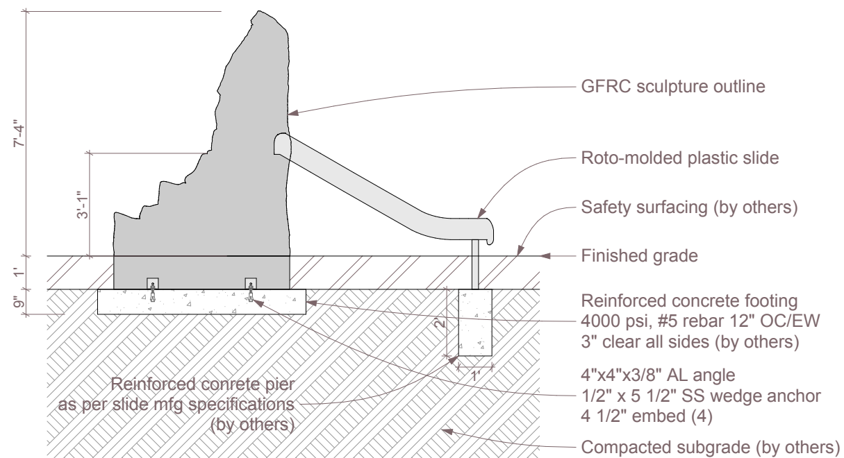
Section SCALE: 1/4" = 1'-0"
