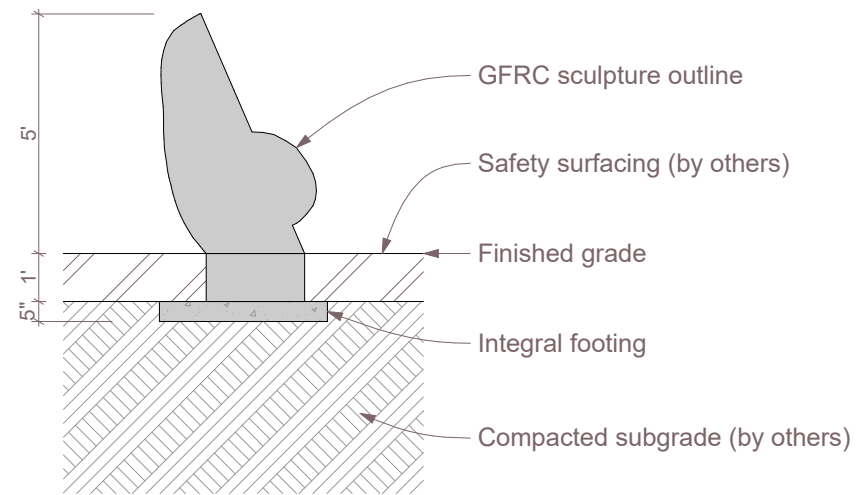
1 Section SCALE: 1/4" = 1'-0"
